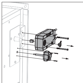
Type BFL(T) sur CR2/CU2/ CU4/CU2-15:
