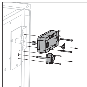
Type BFL(T) op CR2/CU2/ CU4/CU2-15:
