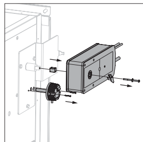
Type BLF(T) sur CR2/CU2/CU4/CU2-15:
